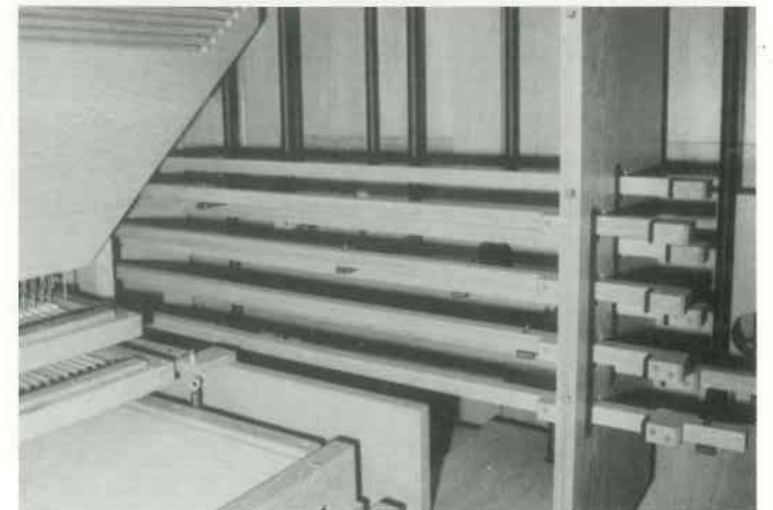
einarmige Tasten, hängende Traktur mit Ausgleich, Registerzüge
