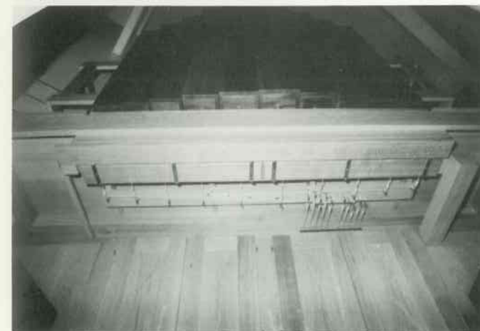
abgeführter Subbaß 16' (Pedal) mit eigener Lade und Traktur
